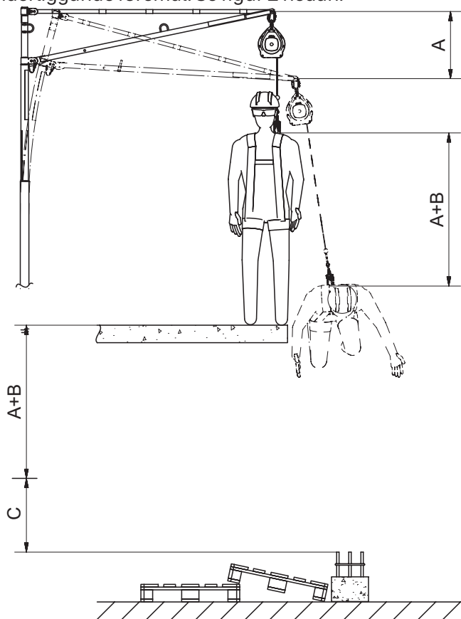
Figur 2. Förklaring av fri fallhöjd.
