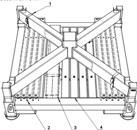
Figur 35. Lastningssystem MkII Basenhet i packat läge.
