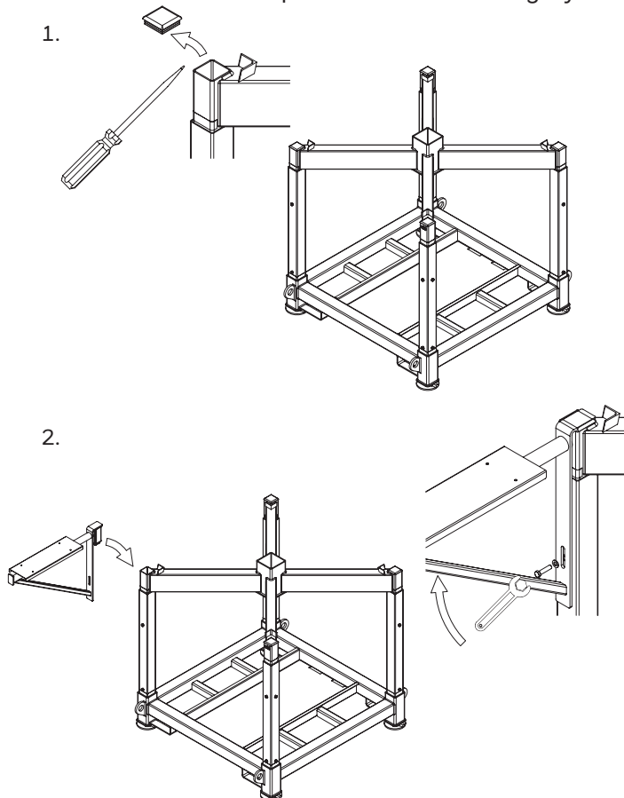
Figur 31. Montera det fasta fästet 8890 på 8800 Lastningssystem MkII
