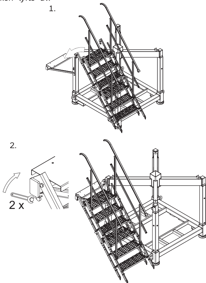
Figur 32. Montera sidotrappan på 8890 trappfäste. Kontrollera UI Site Stairway före installation
