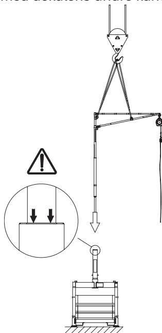
Figur 30. Placering av SkyReach i Toppfylsa 4.7. Var uppmärksam på kranens rörelser för att undvika personskador.
