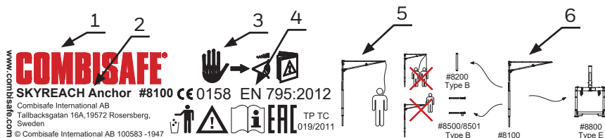
Figur 8. Närbild av dekal med produktinformation
