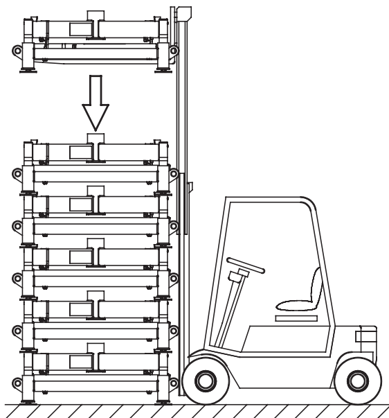
Figur 36. Stapling av den sjätte nedpackade Basenheten på Lastningssystem MkII med gaffeltruck.
