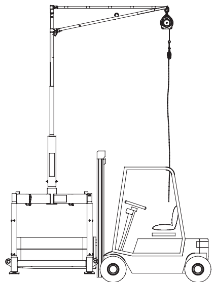
Figur 33. Lyft av komplett enhet vid transport.
