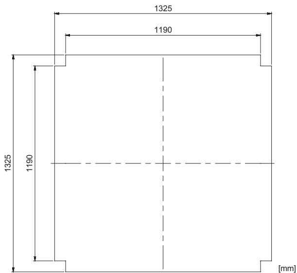
Figur 17. Mått på Bottenskiva.
