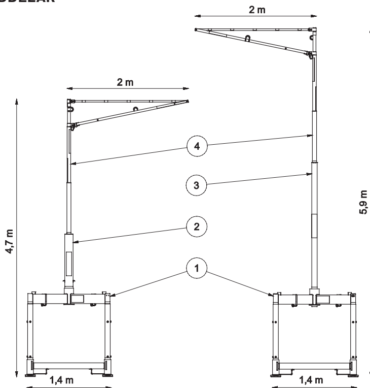
Figur 3. SkyReach Förankringsenhet i monterad och ihopfälld position.
