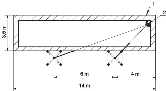
Figur 38. Illustration av arbetsområde vid användning av Dubbelsystem.
