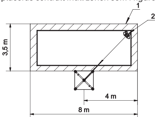
Figur 37. Illustration av arbetsområde vid användning av ett Singelsystem.
